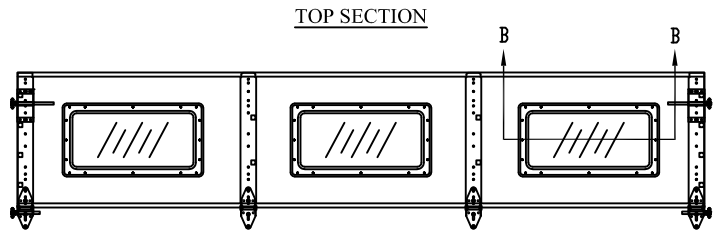
OPTIONAL GLAZED SECTION W/ 24" X 12" WINDOW LAYOUT N.T.S.
