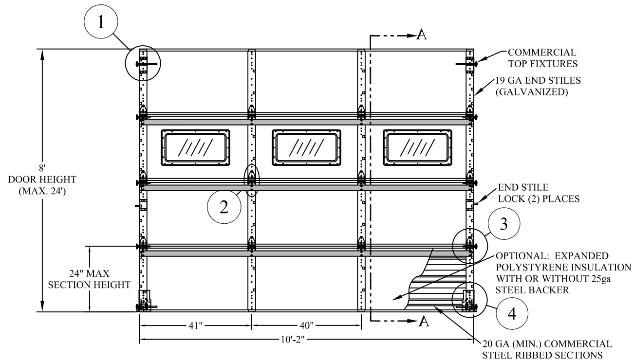
DOOR INTERIOR ELEVATION N.T.S.
